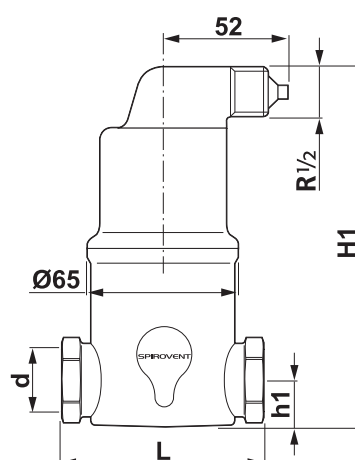
SPIROVENT AA075-AA200
