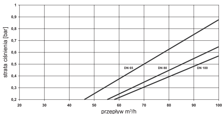
Charakterystyki przepływu dla filtrów flanszowych SYR 6380
